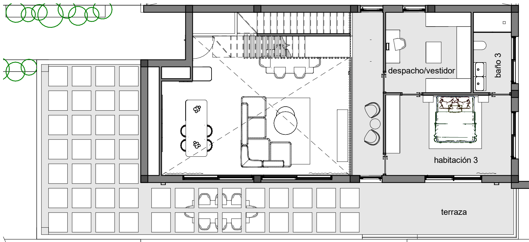
PLANTA PRIMERA
