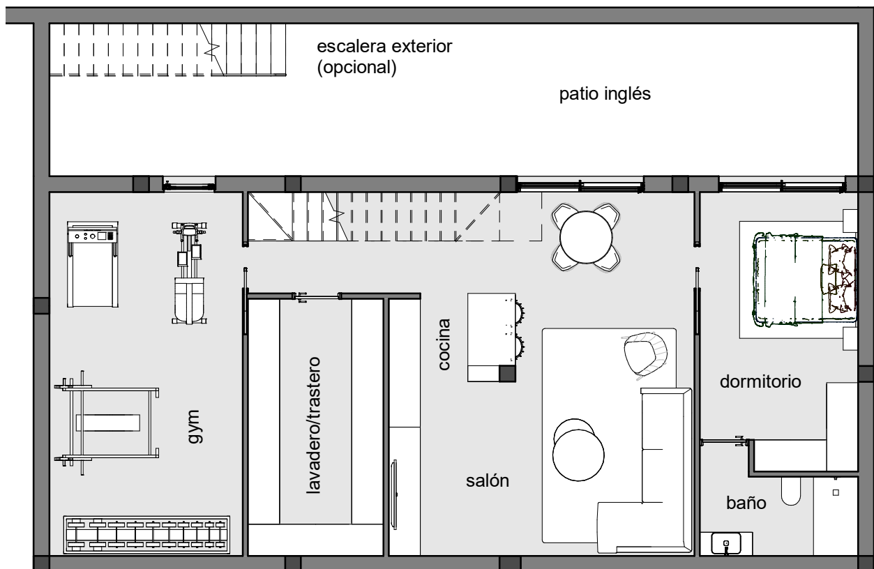
PLANTA SÓTANO (EJEMPLO DE POSIBLE DISTRIBUCIÓN)
